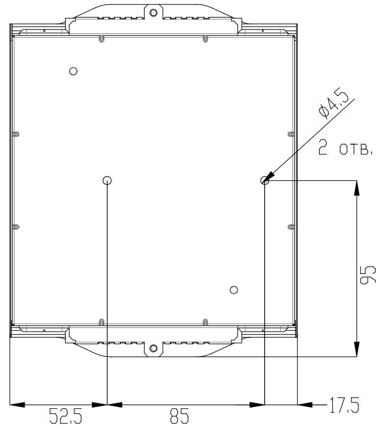
Расположение крепежных отверстий
